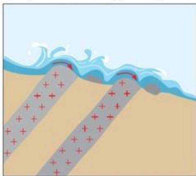
Рис. 74. Схема порогов
