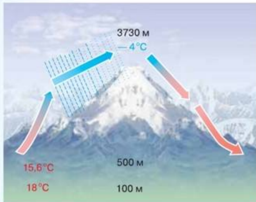
Рис. 97. Насыщенный влагой воздух пересекает горы
