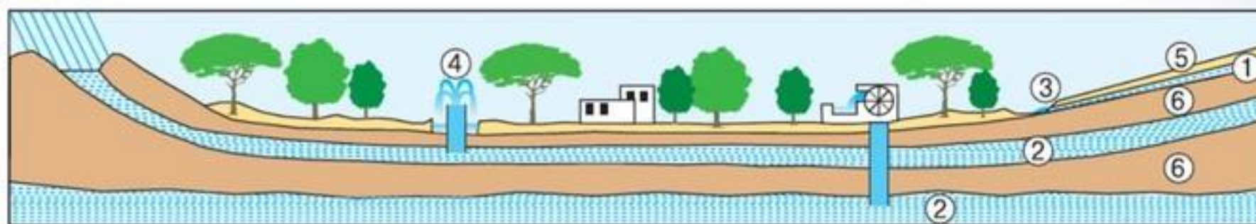
Рис. 79. Подземные воды: 1 — грунтовые воды; 2 — межпластовые воды; 3 — родник; 4 — артезианский источник; 5 — водопроницаемые породы; 6 — водоупорные породы
