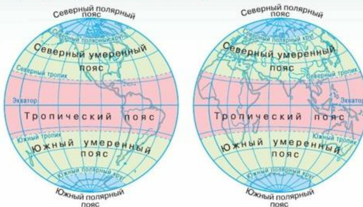
Рис. 17. Пояса освещённости
