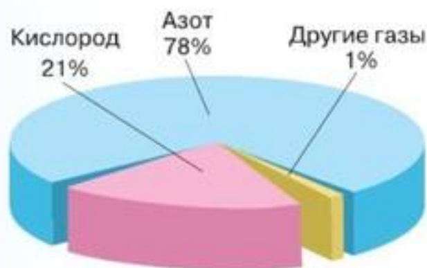
Рис. 83. Состав воздуха
