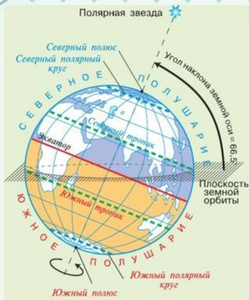
Рис. 15. Схематическое изображение земного шара
