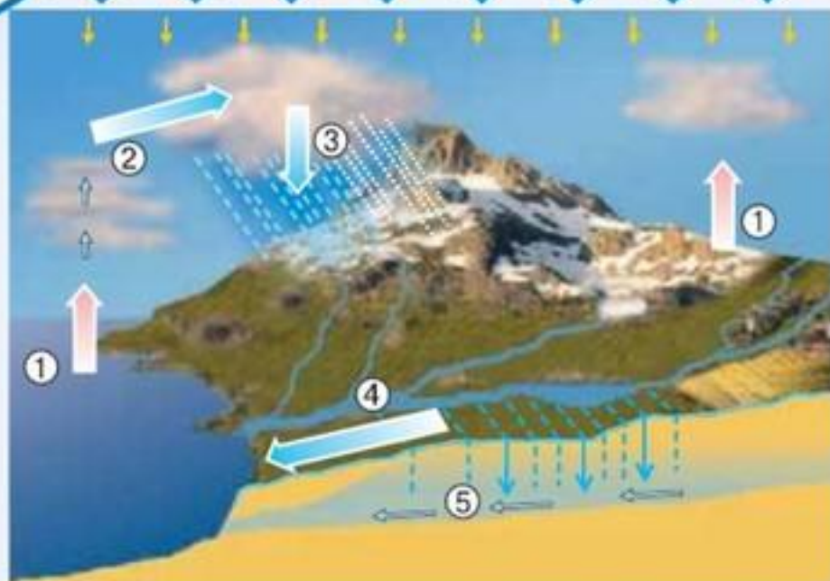
Рис. 60. Мировой круговорот воды:
