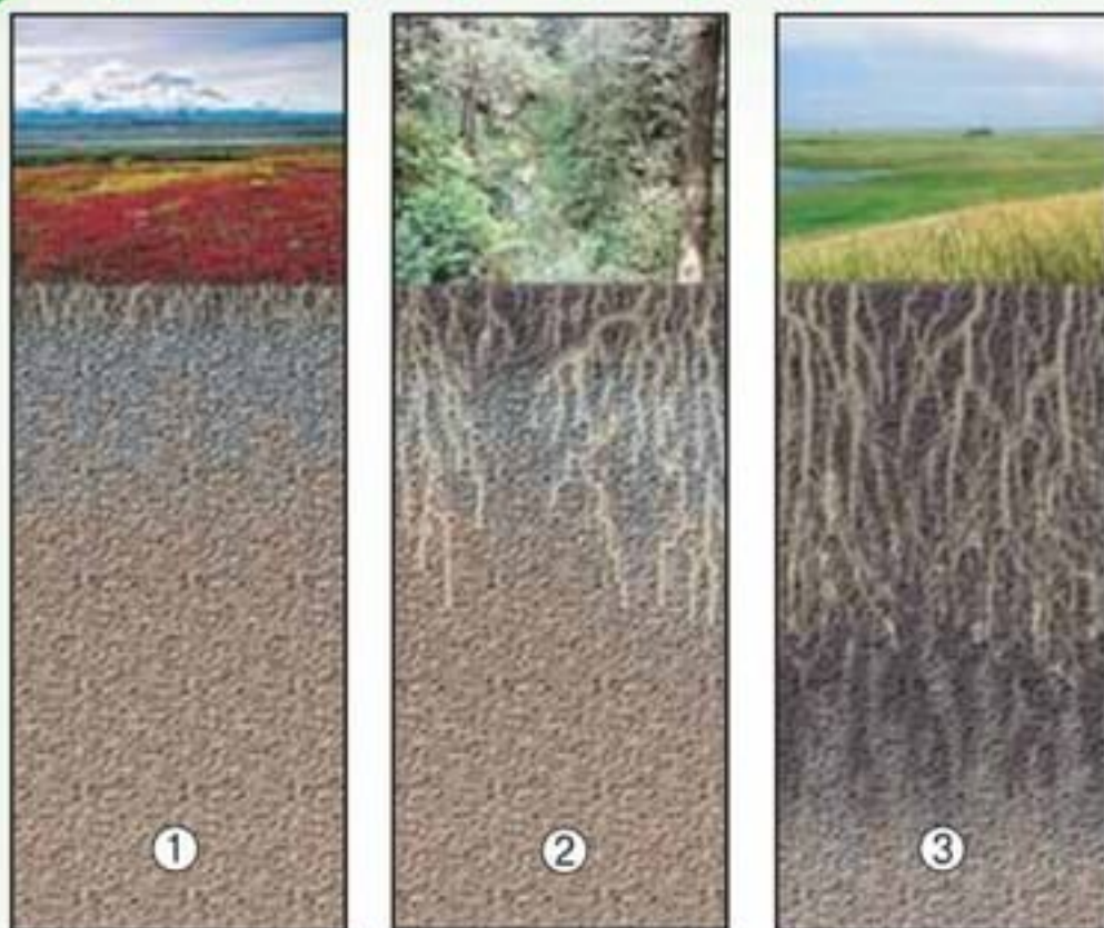
Рис. 108. Типы почв: 1 — тундровая глеевая; 2 — таёжная подзолистая; 3 — чернозём
