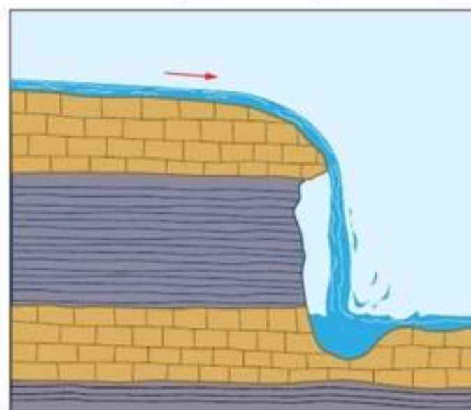
Рис. 75. Схема водопада
