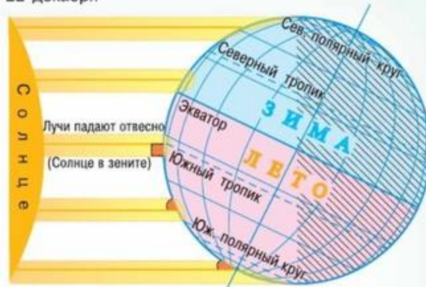
Рис. 19. День зимнего солнцестояния Северного полушария
